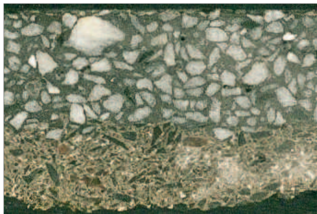
Obr. 8-11: Dvouvrstvý umělý kámen náhrobku MÖCHEL s větším podílem čediče ve spodní desce a mramoru v horní desce. Šířka zobrazení: 3 cm. / Zweilagig aufgebauter Kunststein des Grabmals MÖCHEL mit einem höheren Anteil an Basalt in der unteren und Marmor in der oberen Lage. Bildbreite: 3 cm.
